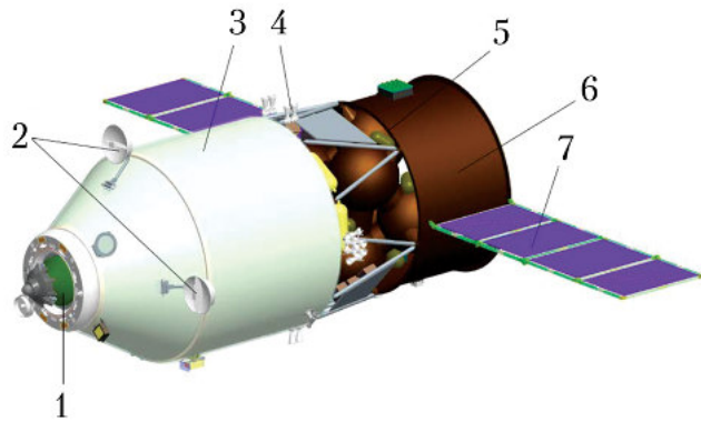
Рис. 4. Транспортный грузовой корабль повышенной грузоподъемности: 1 – стыковочный агрегат; 2 – антенны системы «Курс НА»; 3 – герметичный грузовой отсек; 4 – двигатели ориентации и ориентации (28 шт.); 5 – негерметичный приборно-агрегатный отсек; 6 – радиатор системы обеспечения температурного режима; 7 – панели солнечных батарей
