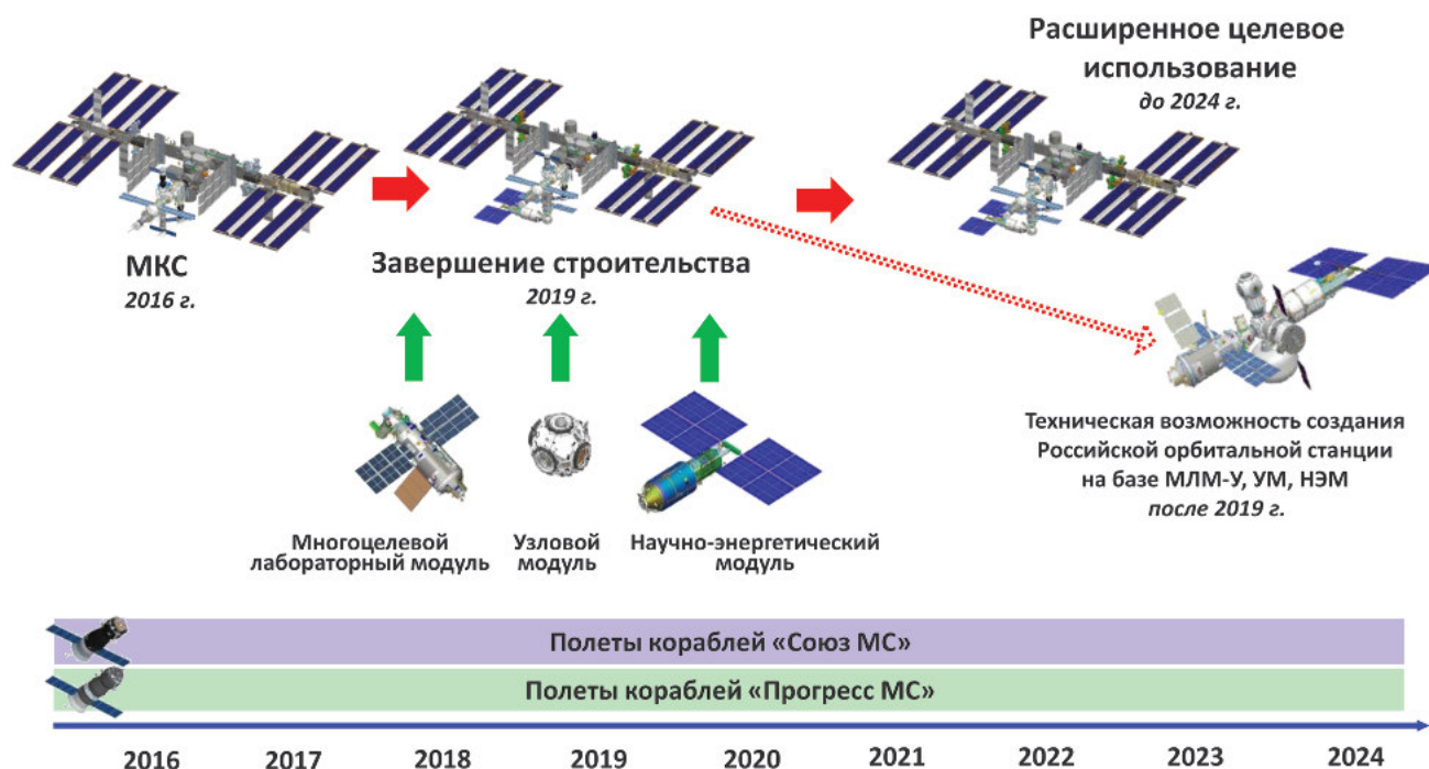
Рис. 2. Строительство Российского сегмента МКС после 2016 г.
